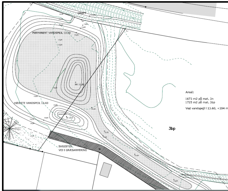
Figur 2: Placering af regnvandsbassin på matr. 3n og 3bp
